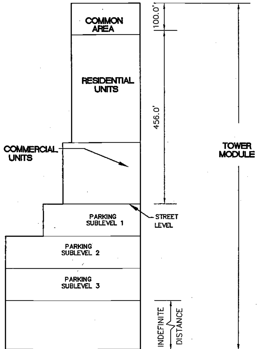
SECTION B-B' N.T.S
